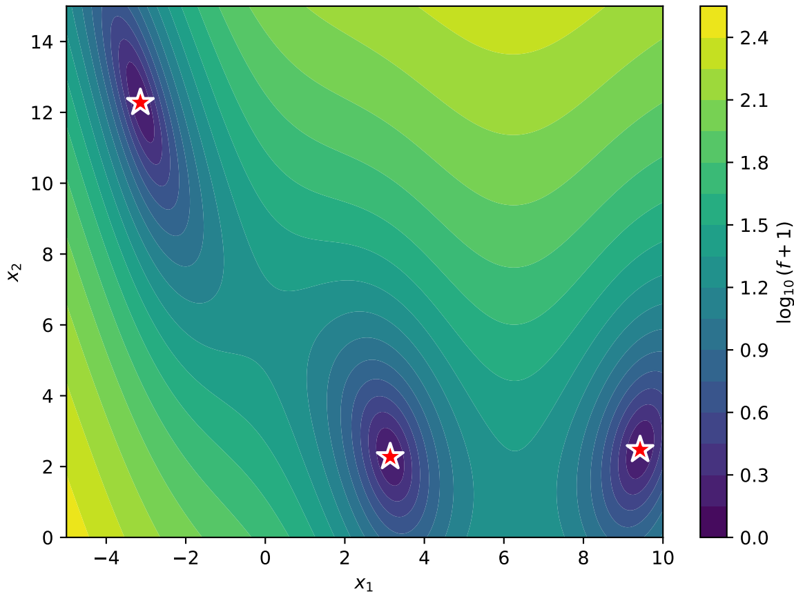
Функція Бренін: \log_{10}(f + 1) і три глобальні мінімуми
